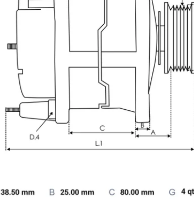
DIMENSIONS
