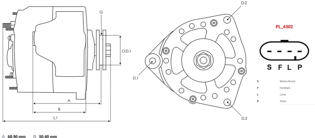
DIMENSIONS
