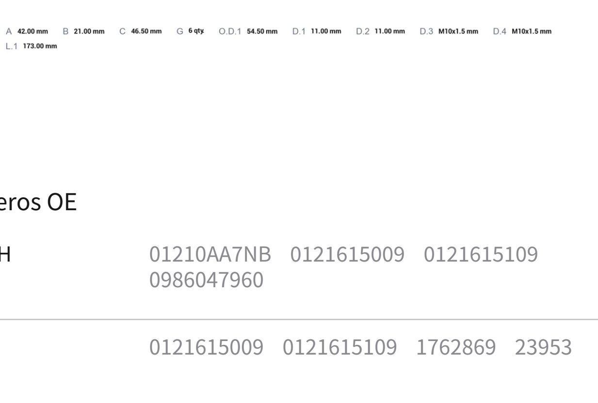
DIMENSIONS
