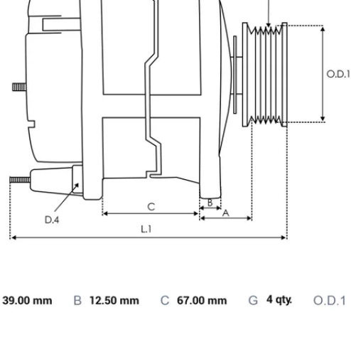
DIMENSIONS
