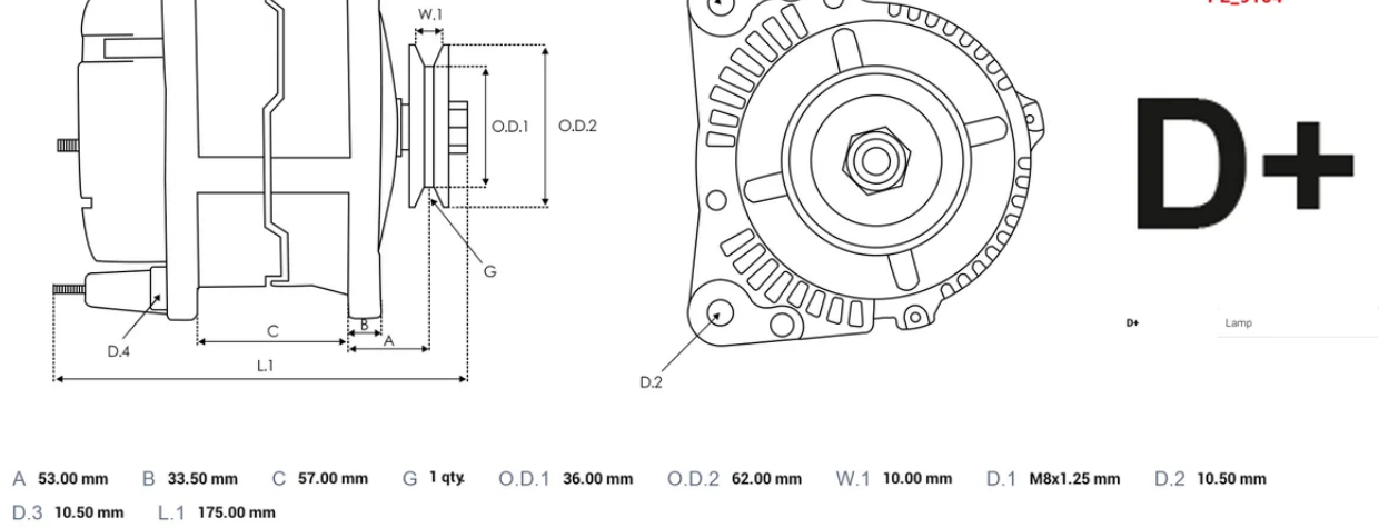
DIMENSIONS
