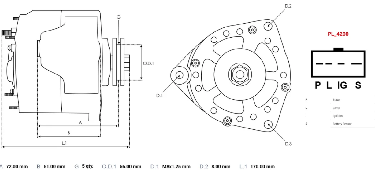
DIMENSIONS
