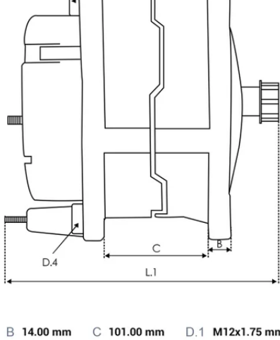
DIMENSIONS
