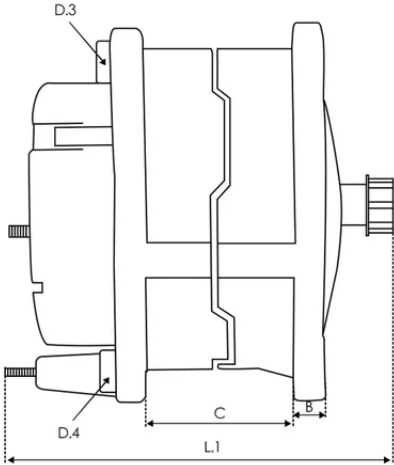
DIMENSIONS
