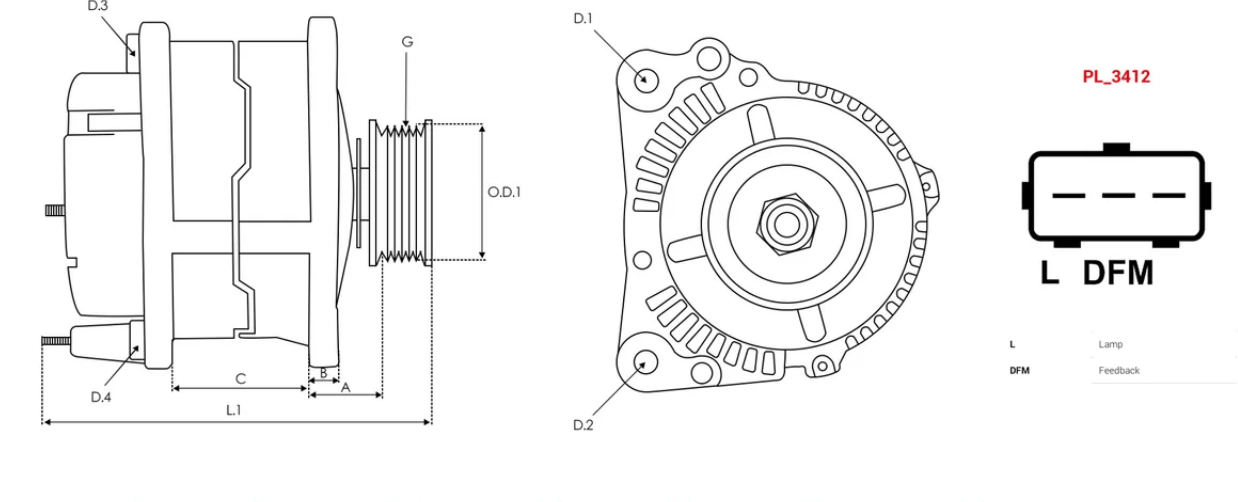
DIMENSIONS
