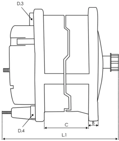
DIMENSIONS
