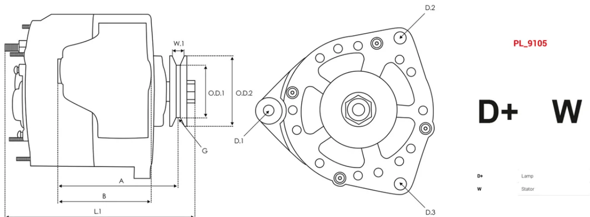
DIMENSIONS
