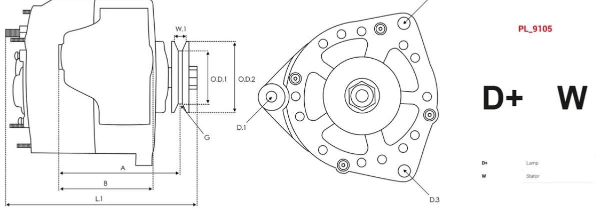
DIMENSIONS
