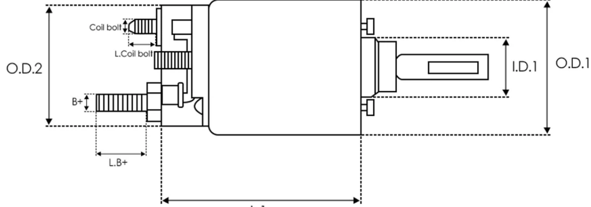
DIMENSIONS
