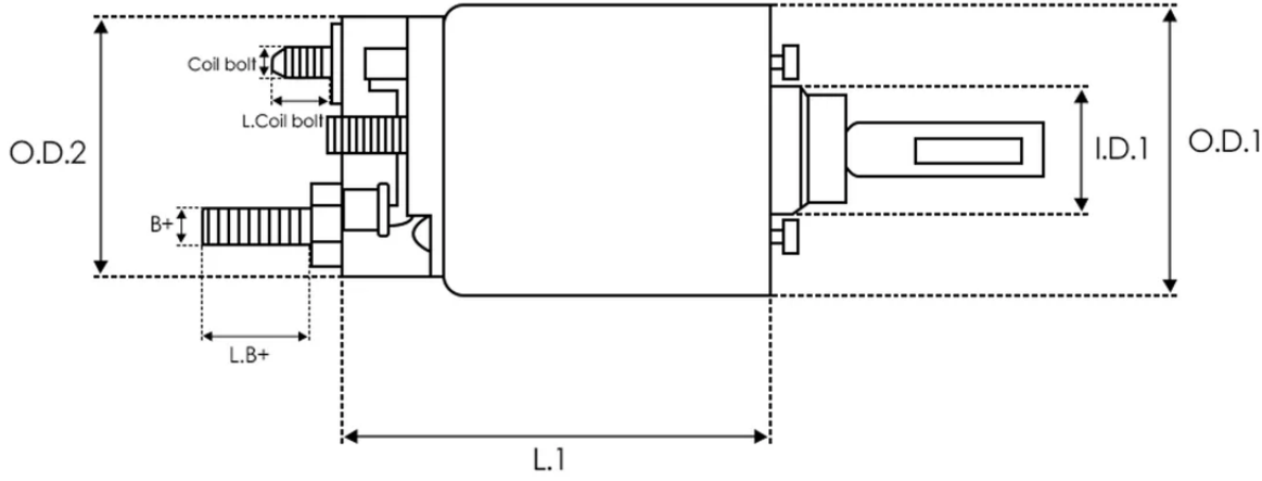
DIMENSIONS
