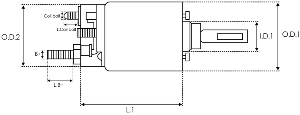
DIMENSIONS
