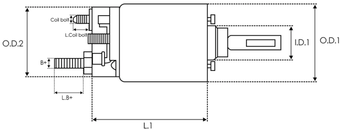
DIMENSIONS
