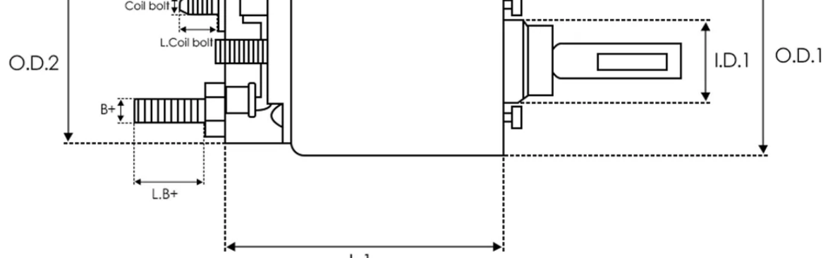
DIMENSIONS
