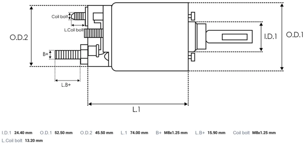
DIMENSIONS
