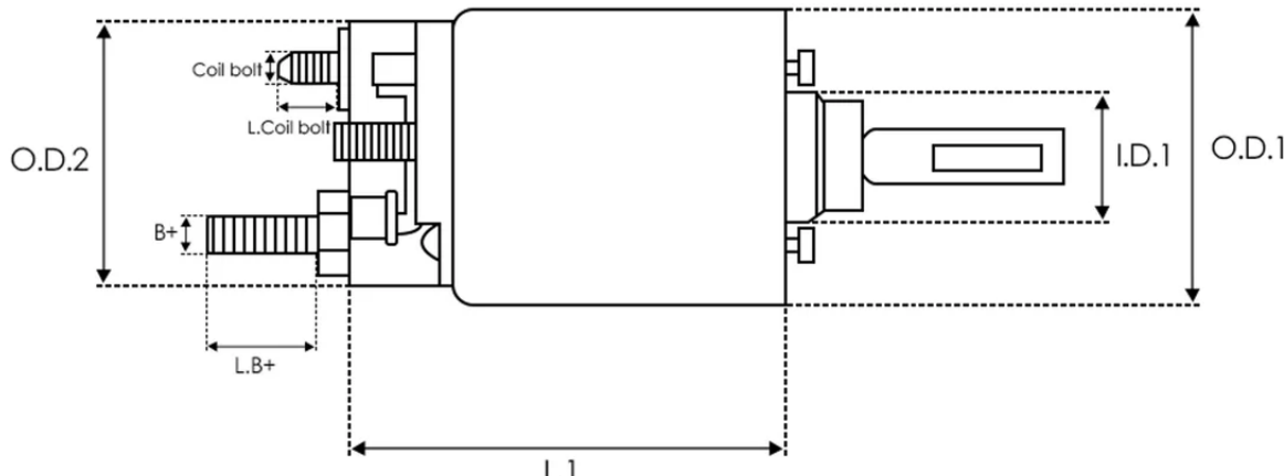
DIMENSIONS
