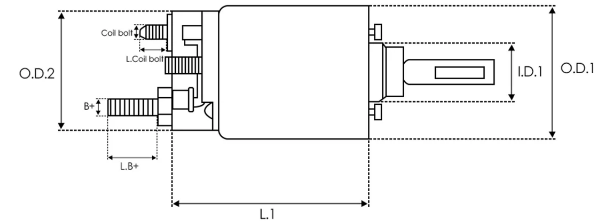
DIMENSIONS
