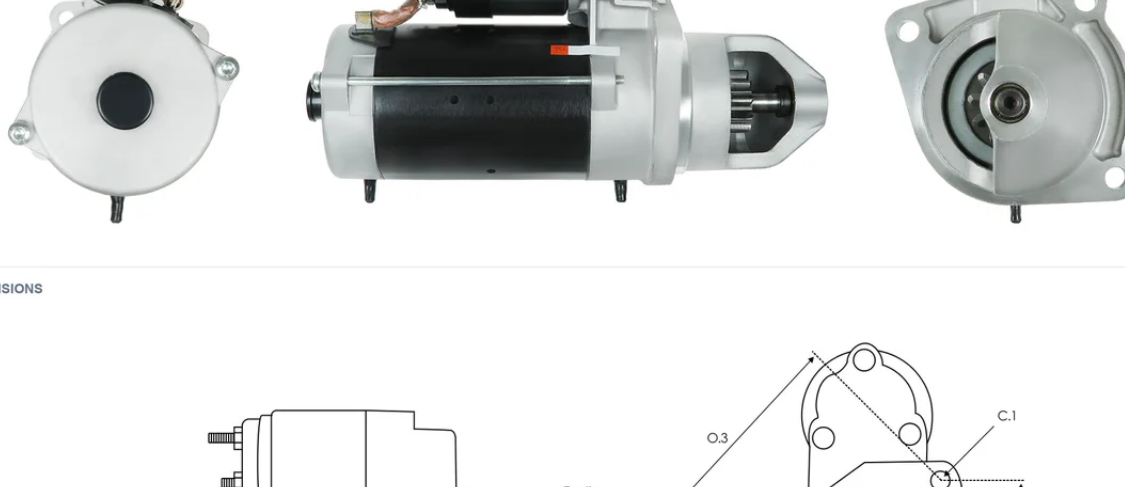
DIMENSIONS
