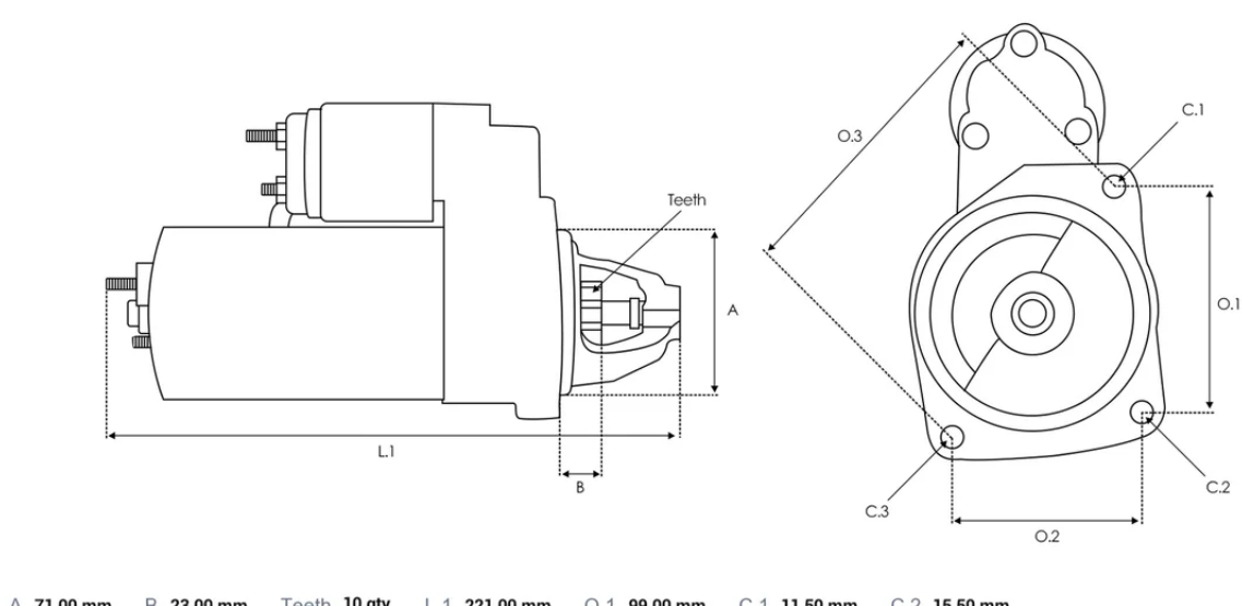
DIMENSIONS
