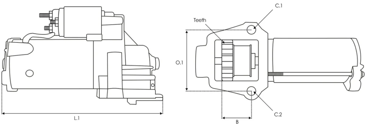
DIMENSIONS
