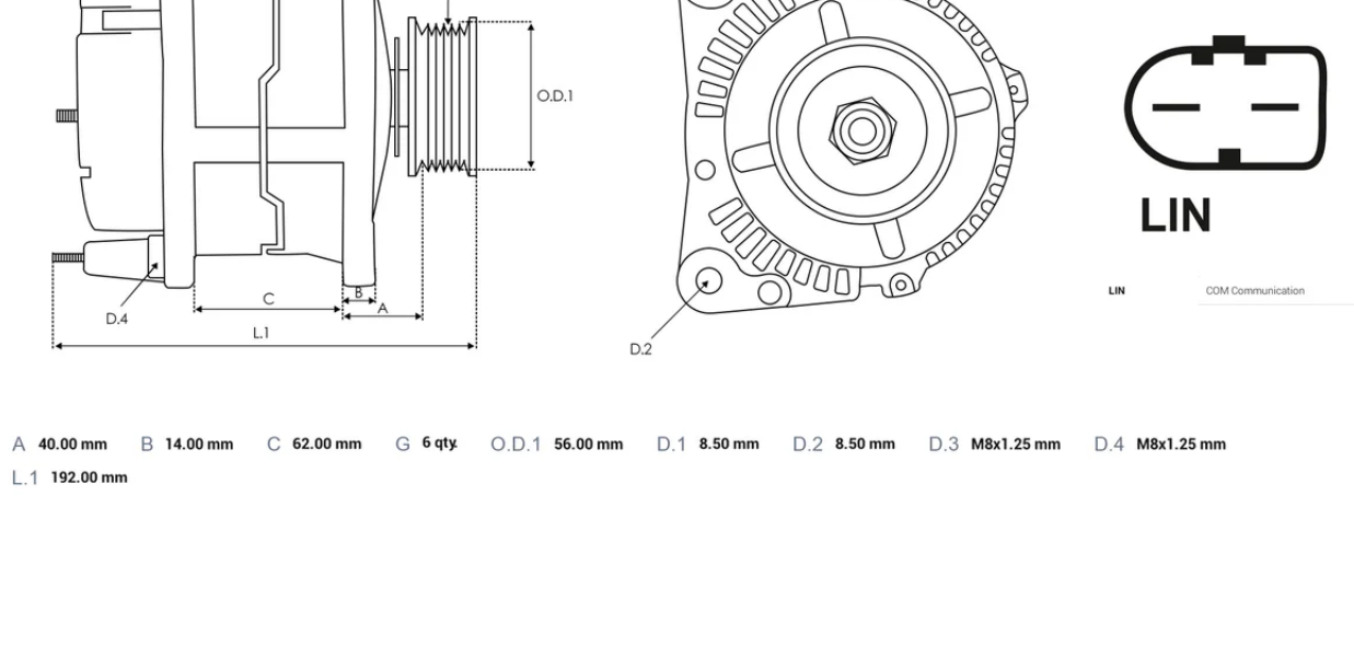
DIMENSIONS
