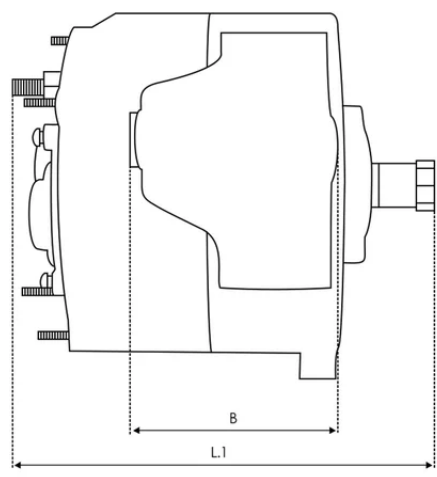
DIMENSIONS
