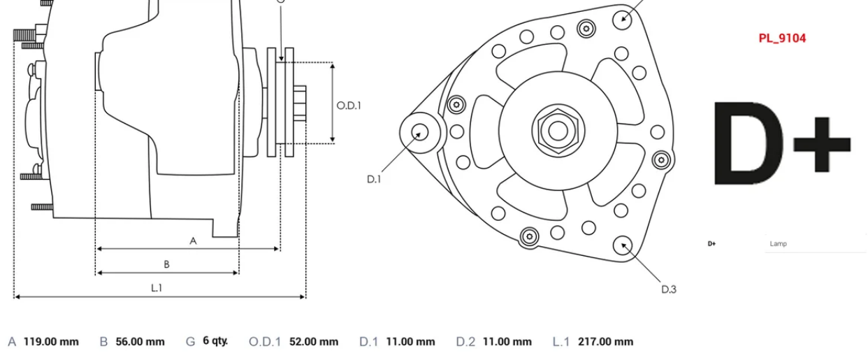
DIMENSIONS
