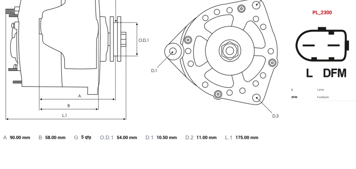
DIMENSIONS
