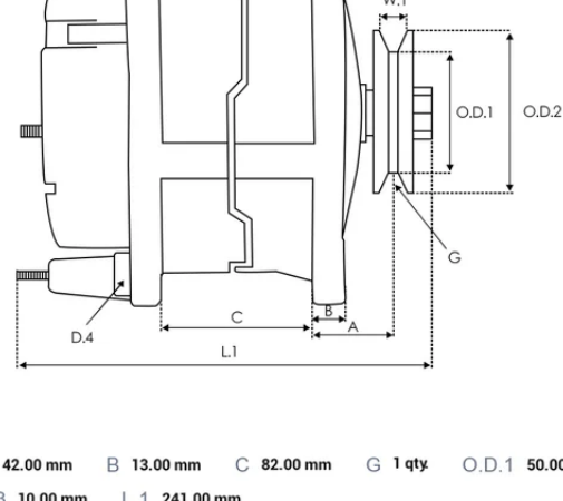
DIMENSIONS
