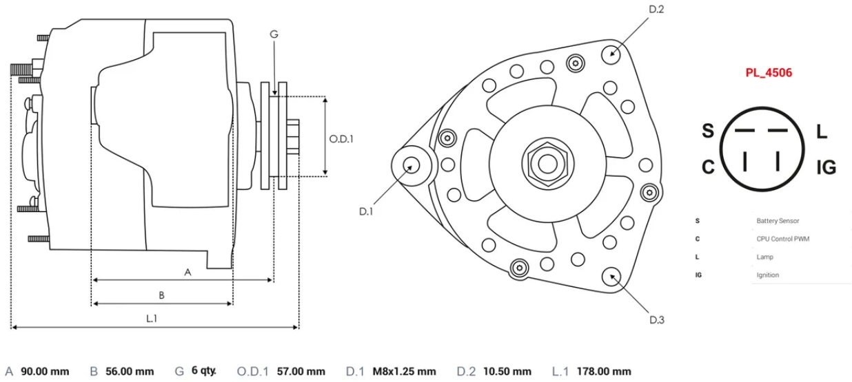
DIMENSIONS
