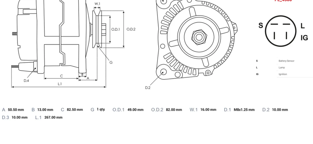
DIMENSIONS
