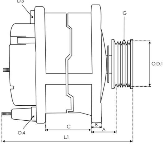
DIMENSIONS
