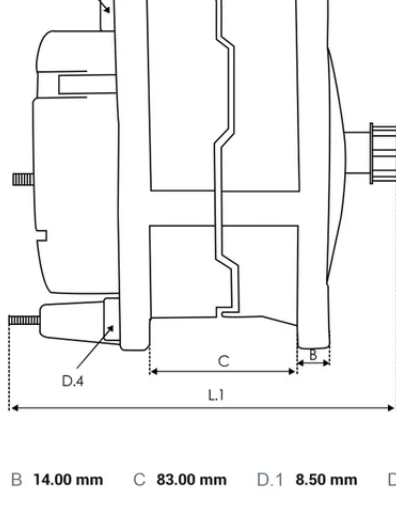
DIMENSIONS
