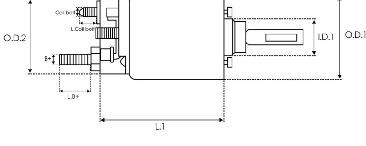
DIMENSIONS
