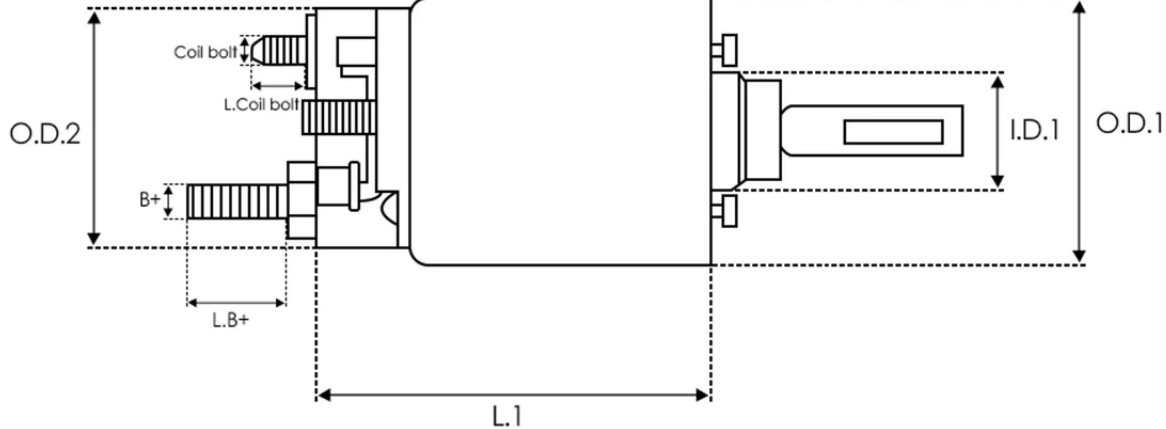
DIMENSIONS
