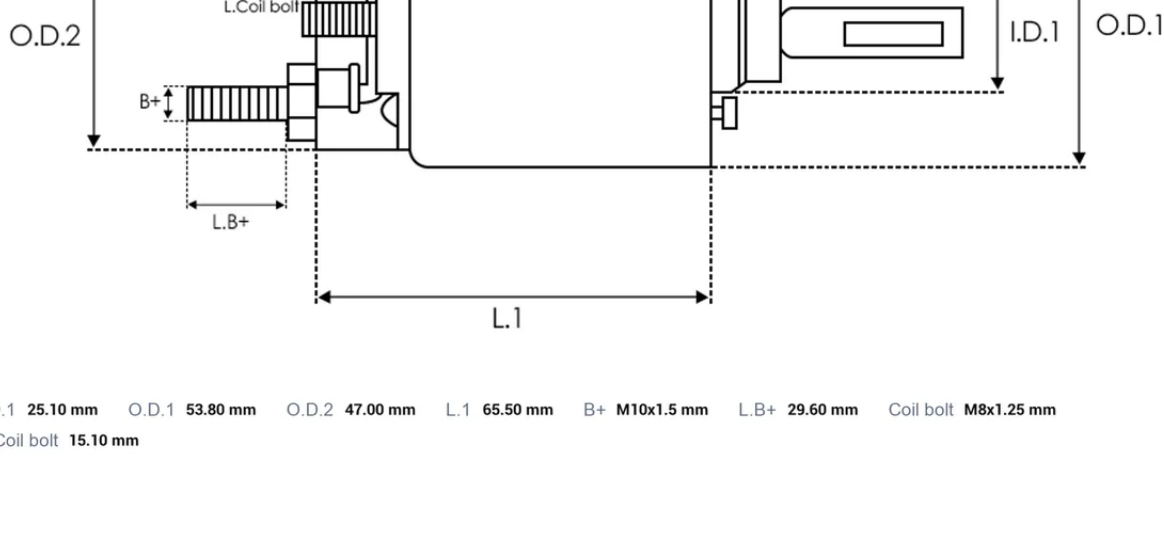
DIMENSIONS
