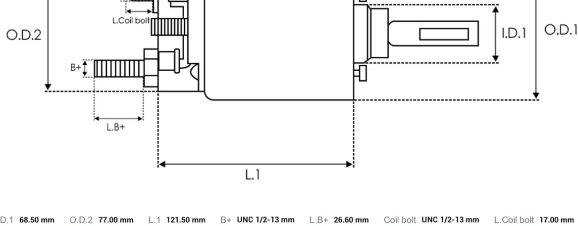
DIMENSIONS
