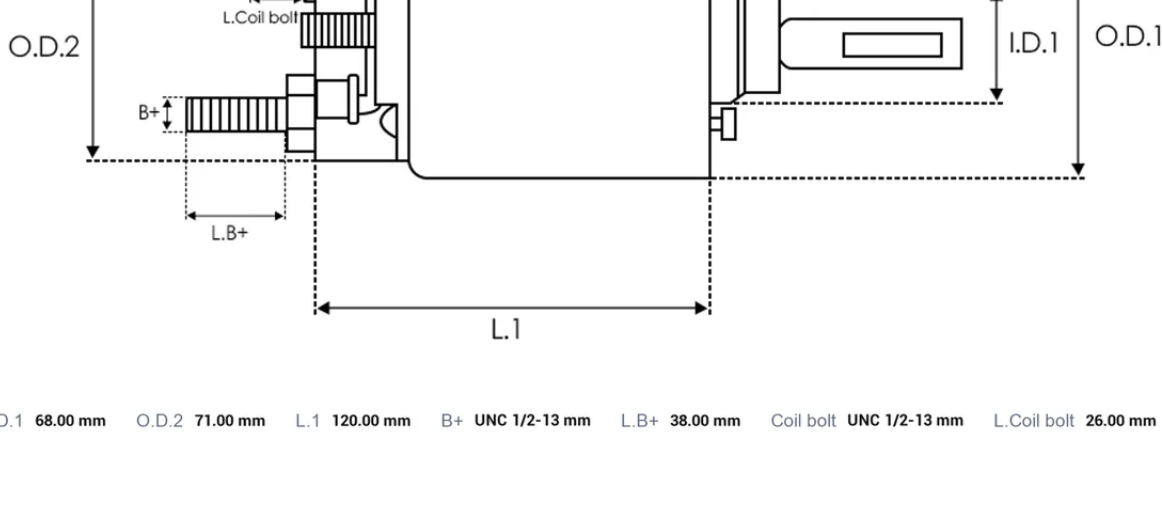
DIMENSIONS
