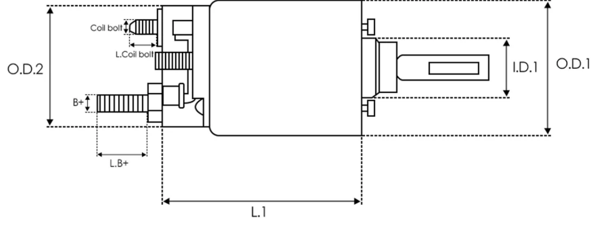
DIMENSIONS
