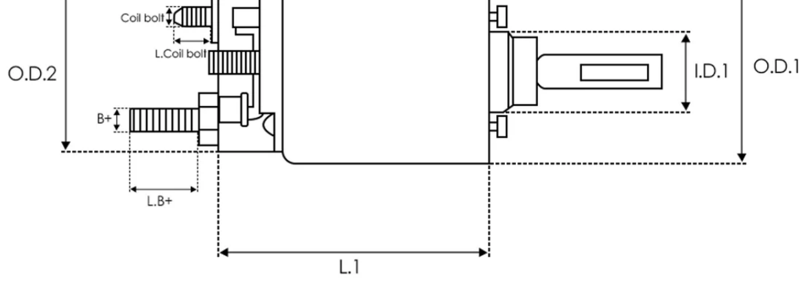
DIMENSIONS
