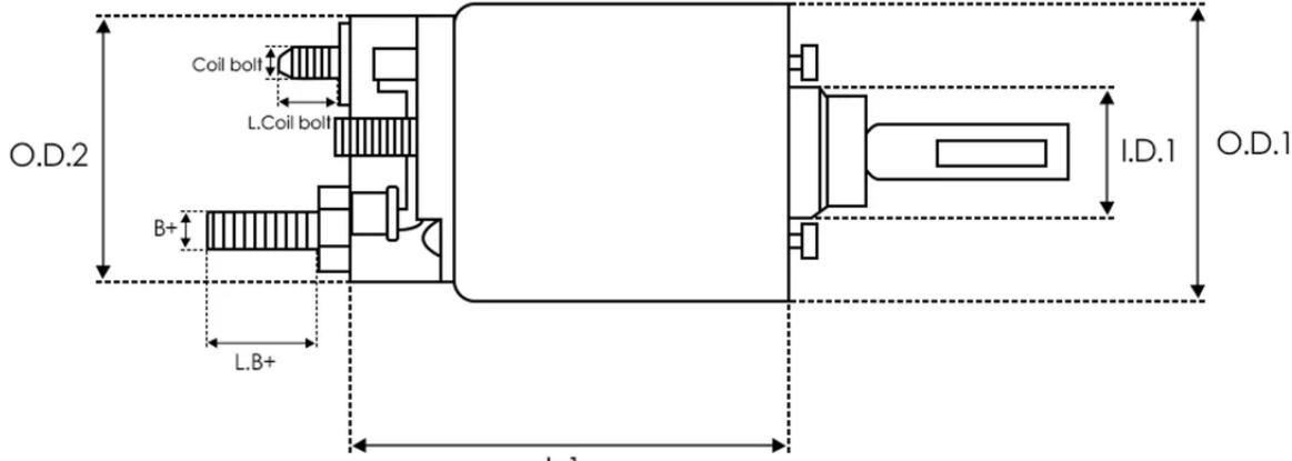
DIMENSIONS
