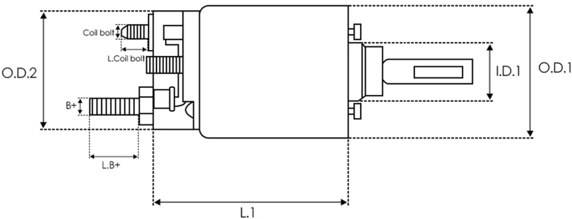
DIMENSIONS
