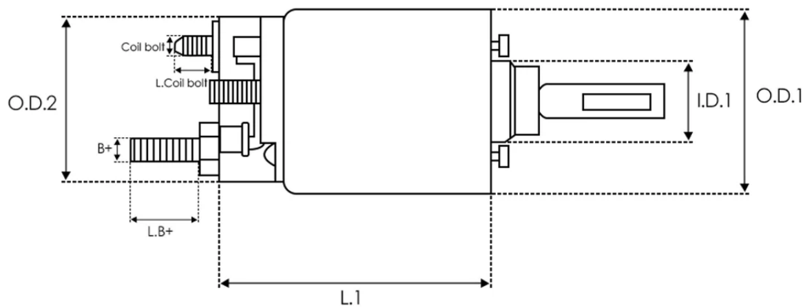
DIMENSIONS
