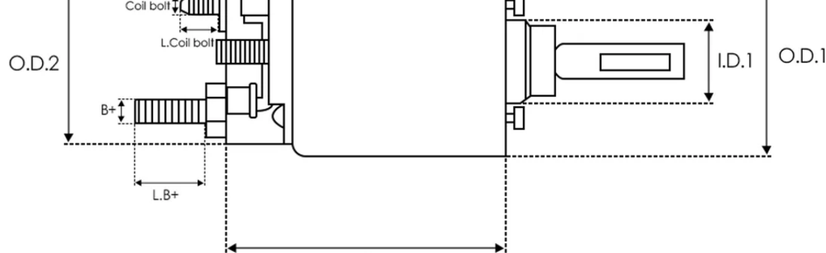
DIMENSIONS
