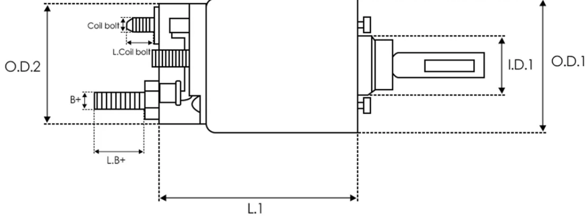
DIMENSIONS
