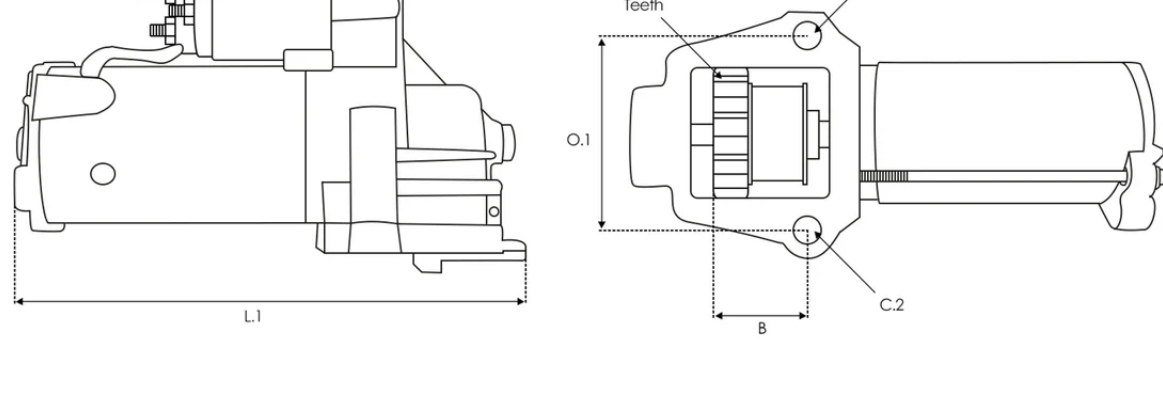
DIMENSIONS
