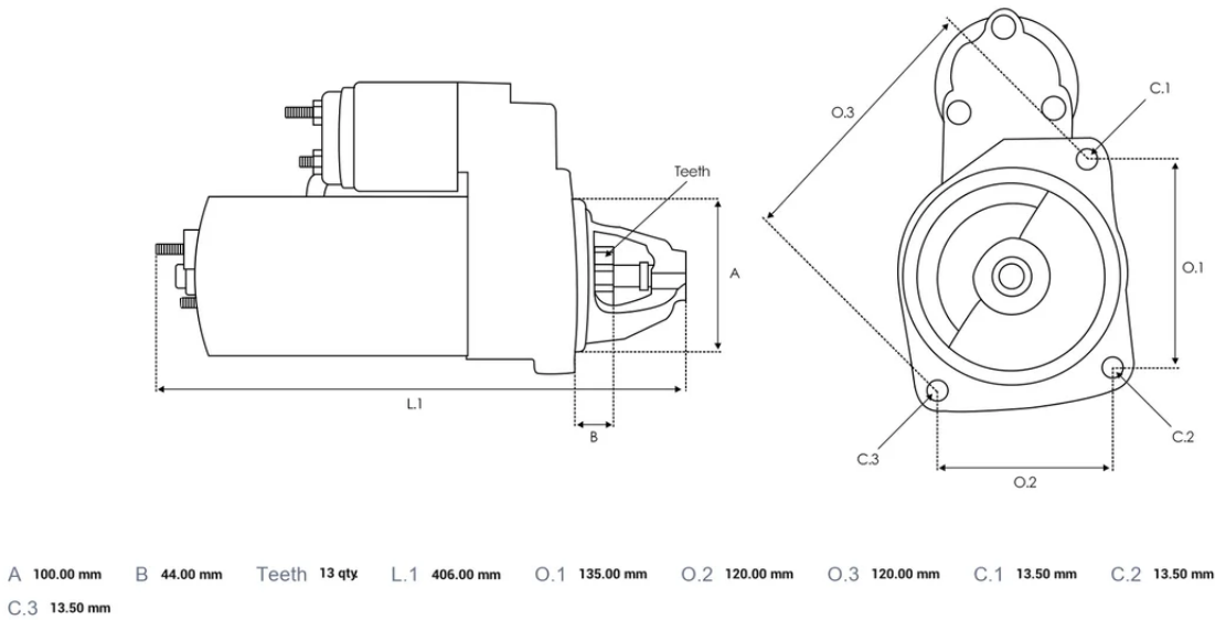
DIMENSIONS
