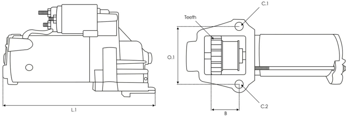
DIMENSIONS
