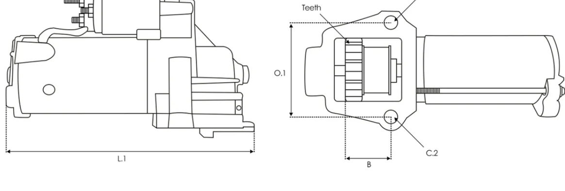
DIMENSIONS
