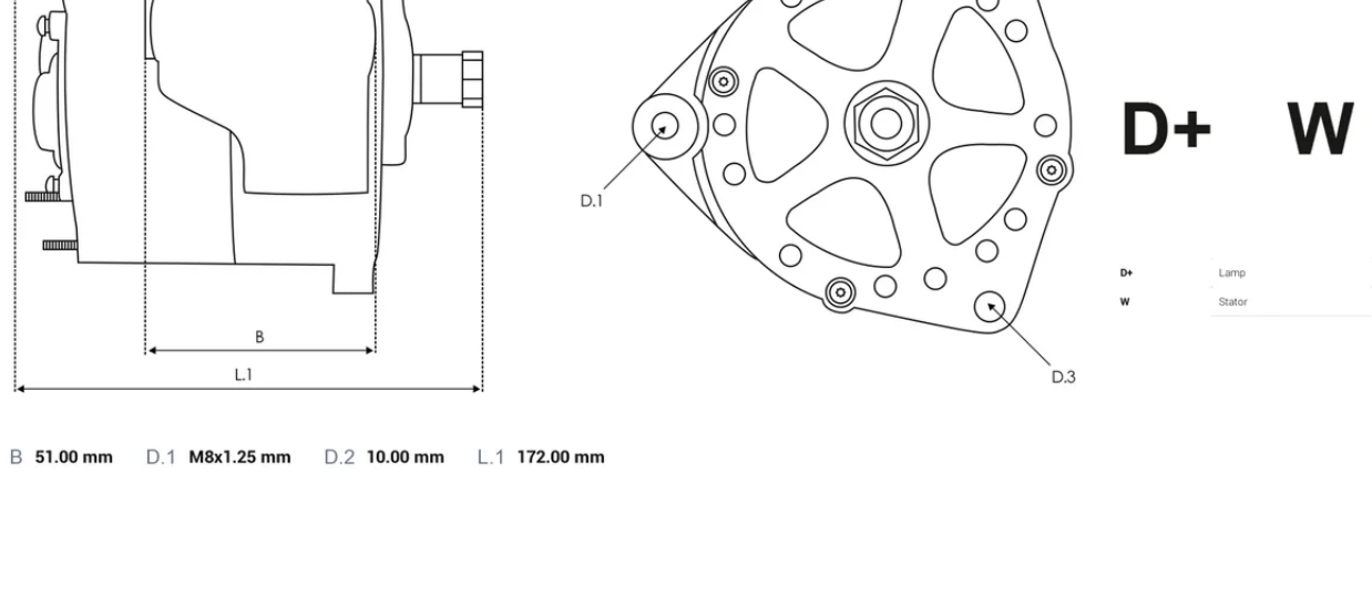
DIMENSIONS
