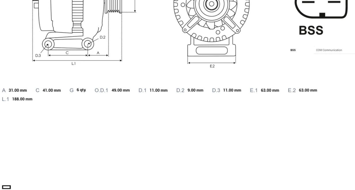
DIMENSIONS
